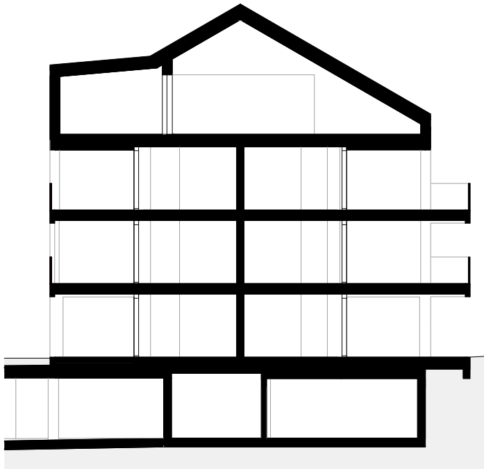
Querschnitt
